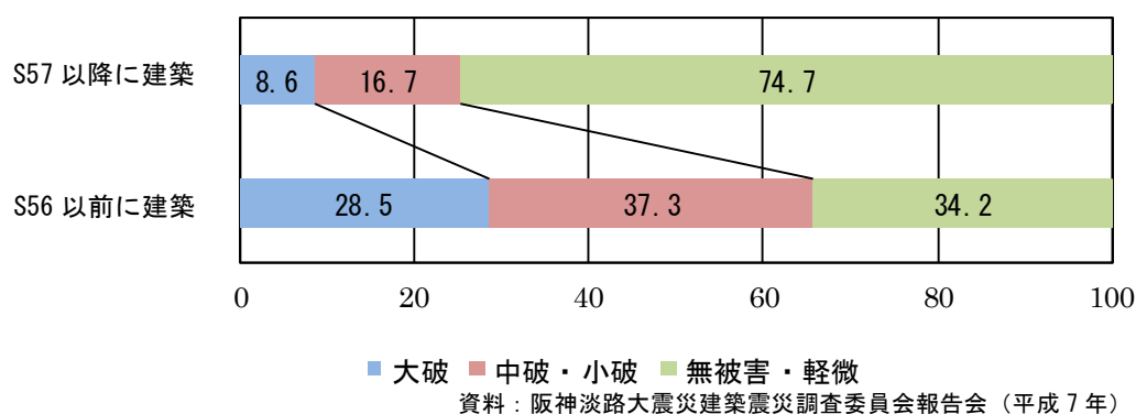
図 2-1：阪神・淡路大震災での建物被害割合
