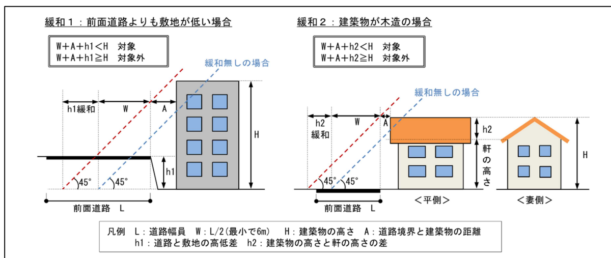
図 6-3：通行障害建築物の要件の緩和
