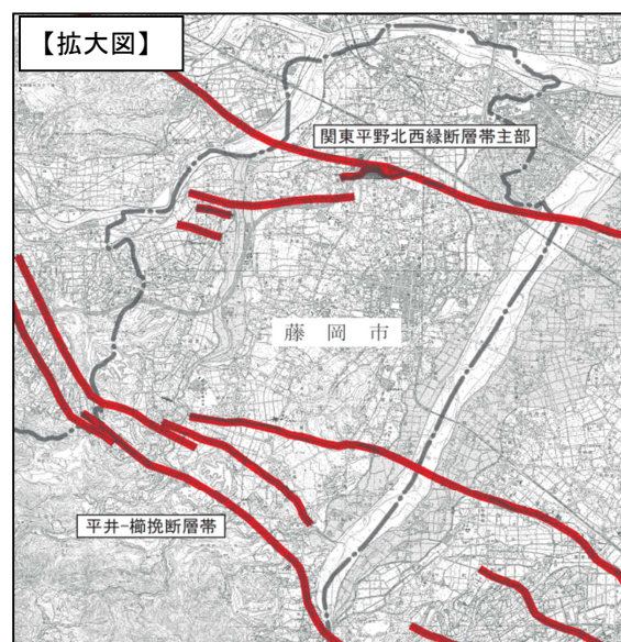
図 3-1：群馬県の構造線・活断層の分布図 (出典：群馬県耐震改修促進計画、国土地理院資料)
