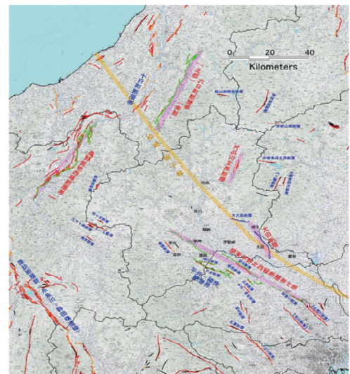
図 3-3：群馬県内の構造線や活断層の分布 (出典：群馬県地震被害想定調査 (H24. 6))
